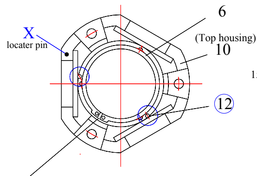
Fig. 3 Section B-B
